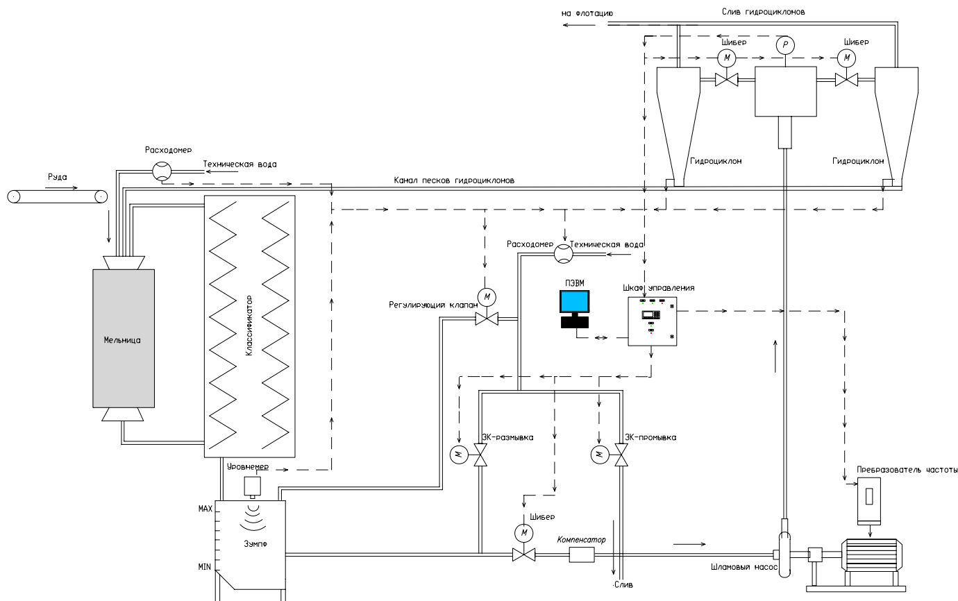
Рис.1 Структурная схема управления установкой классификации рудных пульп.
