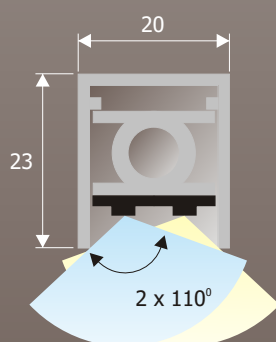
Светильник в разрезе
